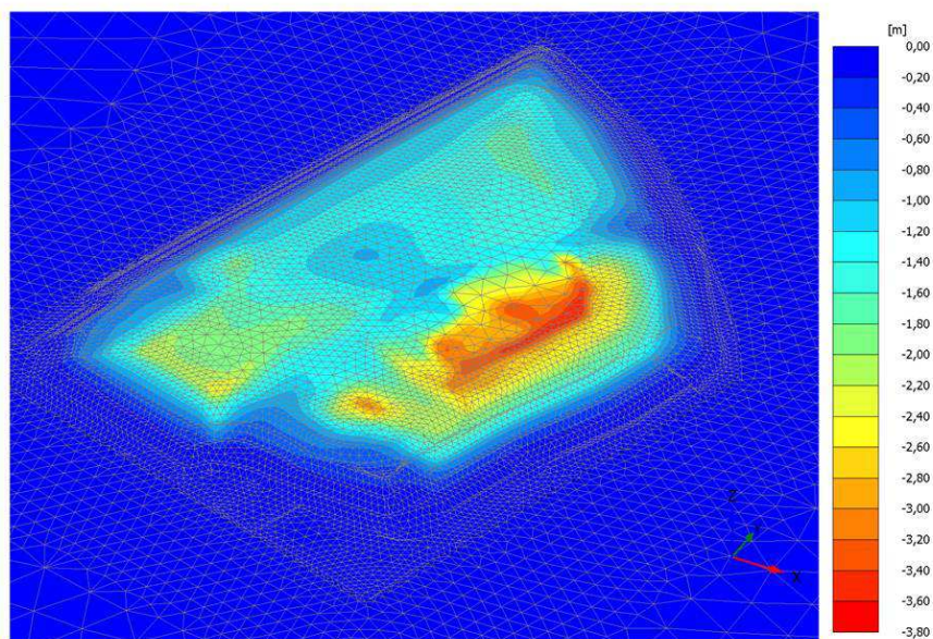
Abb. 7: Setzungen des Deponiekörpers im Endzustand
