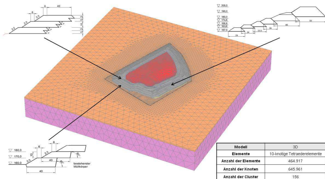
Abb. 5: 3D-FE-Modell der gesamten Deponie im Endzustand mit Darstellung der verschiedenen Randaufbauformen und Angaben zur Anzahl der 3D-Kontinuums-elemente
