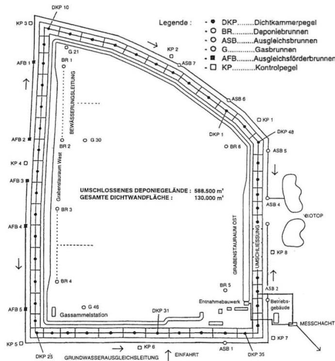
Abb. 1: Schema der vertikalen Deponieumschließung
