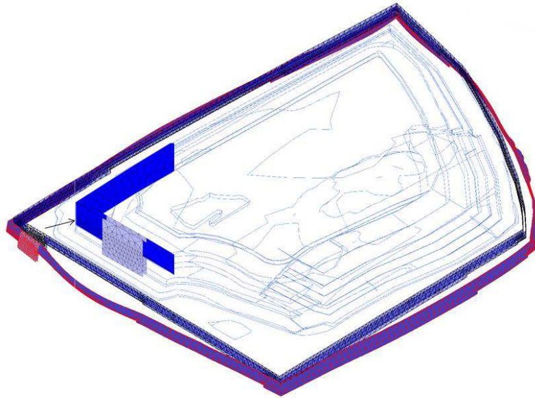
Abb. 6: 3D-FE-Modell des Dichtwandsystems, unverformt und verformt für den Endzustand
